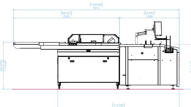
Vue de côté | Velocity MID-TIER 2 postes
