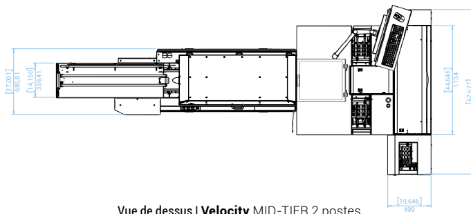
Vue de dessus | Velocity MID-TIER 2 postes
